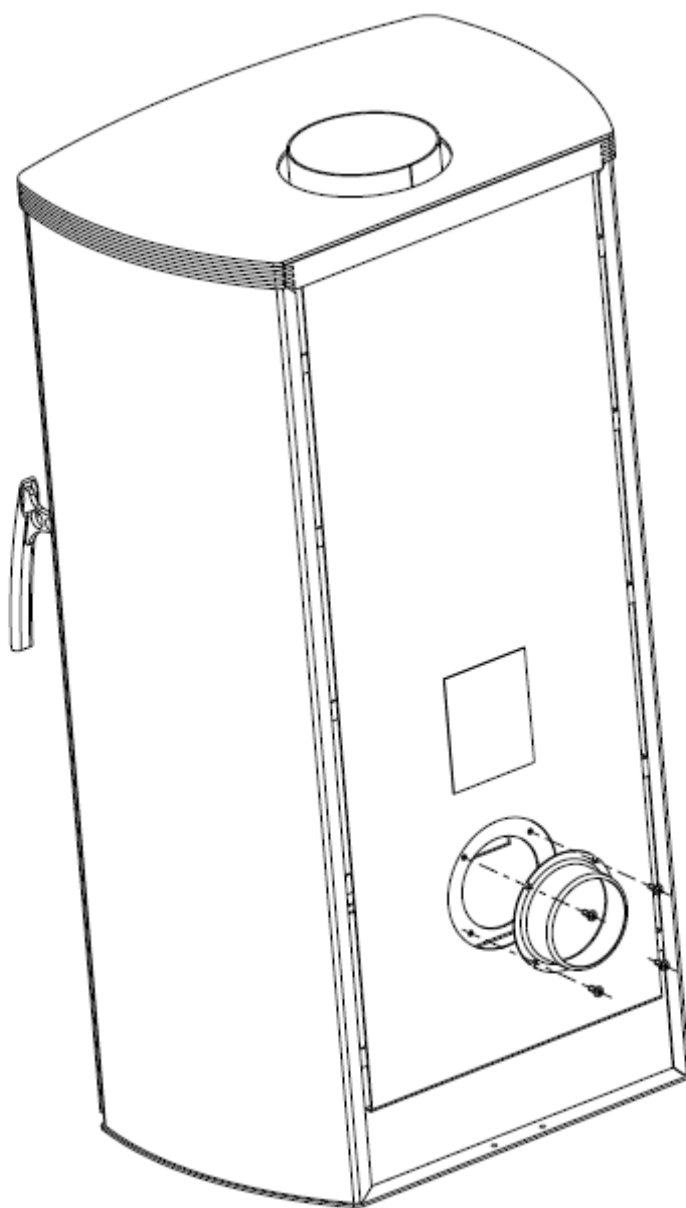
Mainting pipe support for combustion air intake Installation des Stutzens für Anschluss der Verbrennungsluft Inštalácia hrdla pre prívod spaľovacieho vzduchu Instalace hrdla pro přívod spalovacího vzduchu Az égési levegő bevezetésének előkészítése
